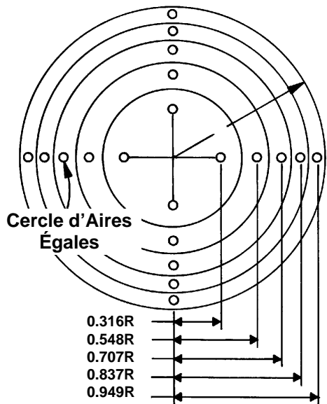
Points de traverses de conduits circulaires
